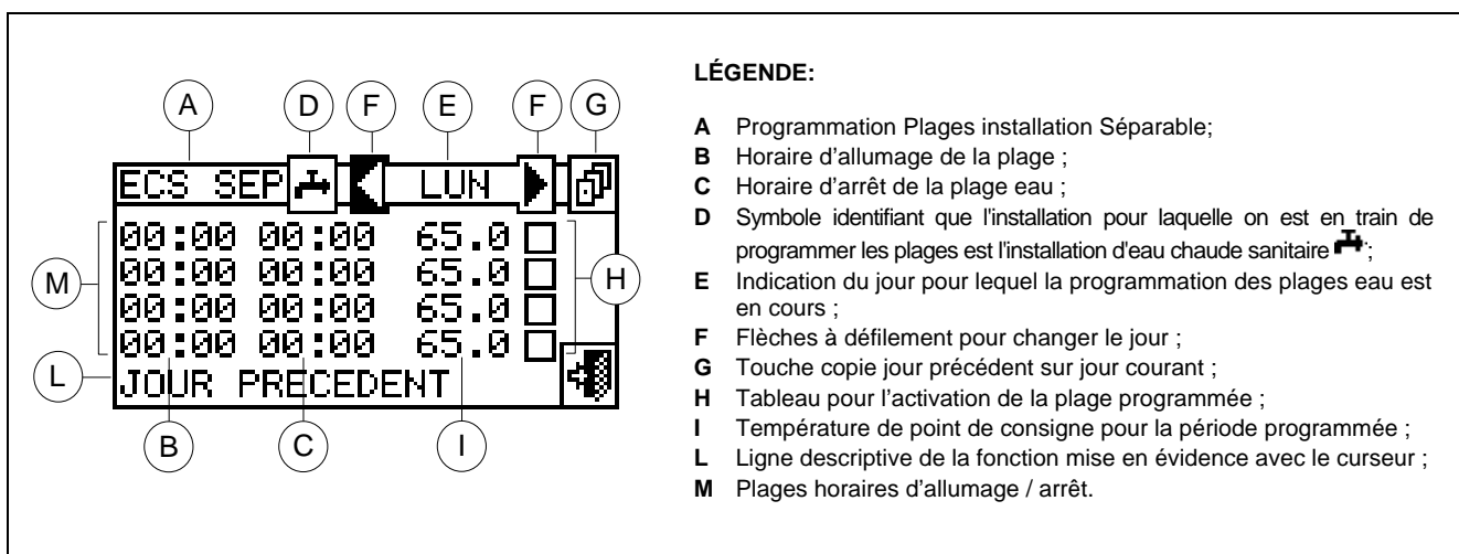
Figure 9 – ECRAN POUR LA PROGRAMMATION DES PLAGES EAU INSTALLATION SEPARABLE
