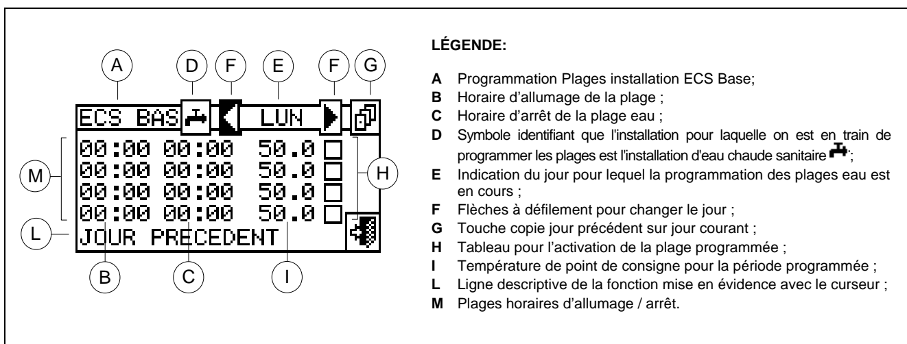
Figure 8 – ECRAN POUR LA PROGRAMMATION DES PLAGES EAU INSTALLATION DE BASE
