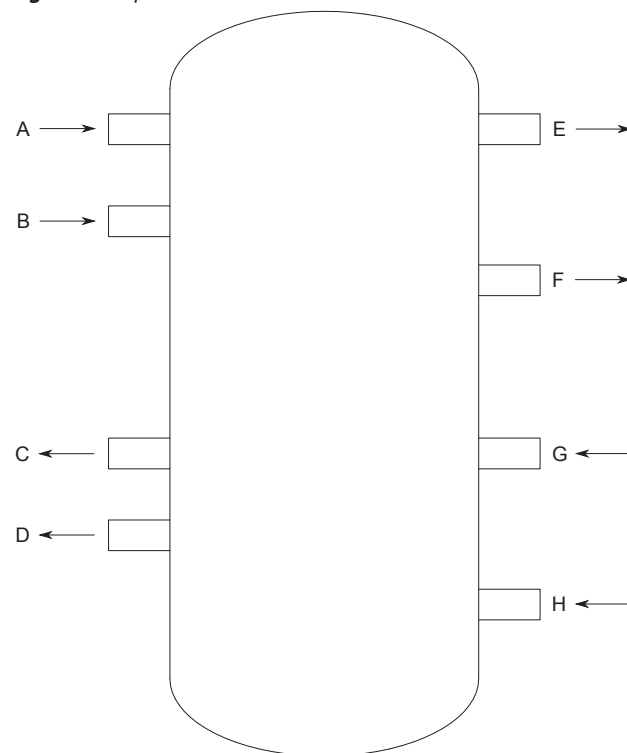
Figura 1.2 Separatore idraulico 8 attacchi
