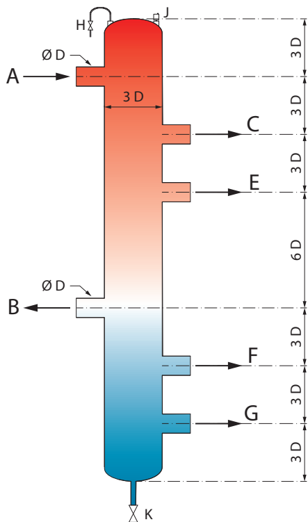
Figura 1.1 Separatore idraulico 6 attacchi
