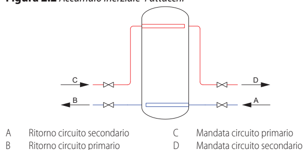
Figura 2.2 Accumulo inerziale 4 attacchi
