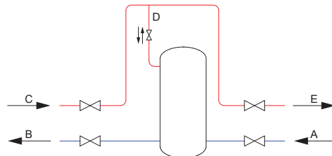
Figura 2.6 Accumulo inerziale 3 attacchi
