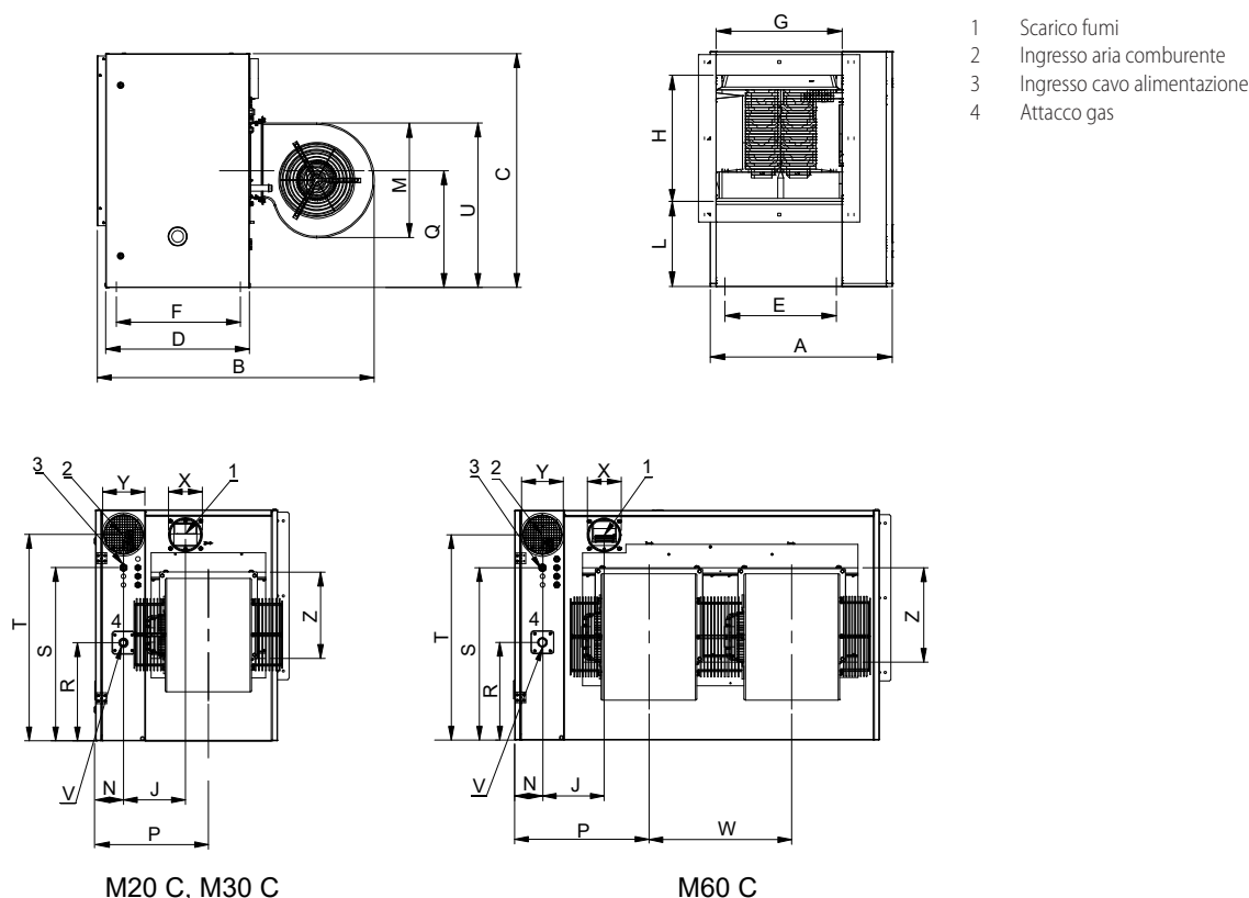
Figura 4.2 Dimensioni generatori serie M C
