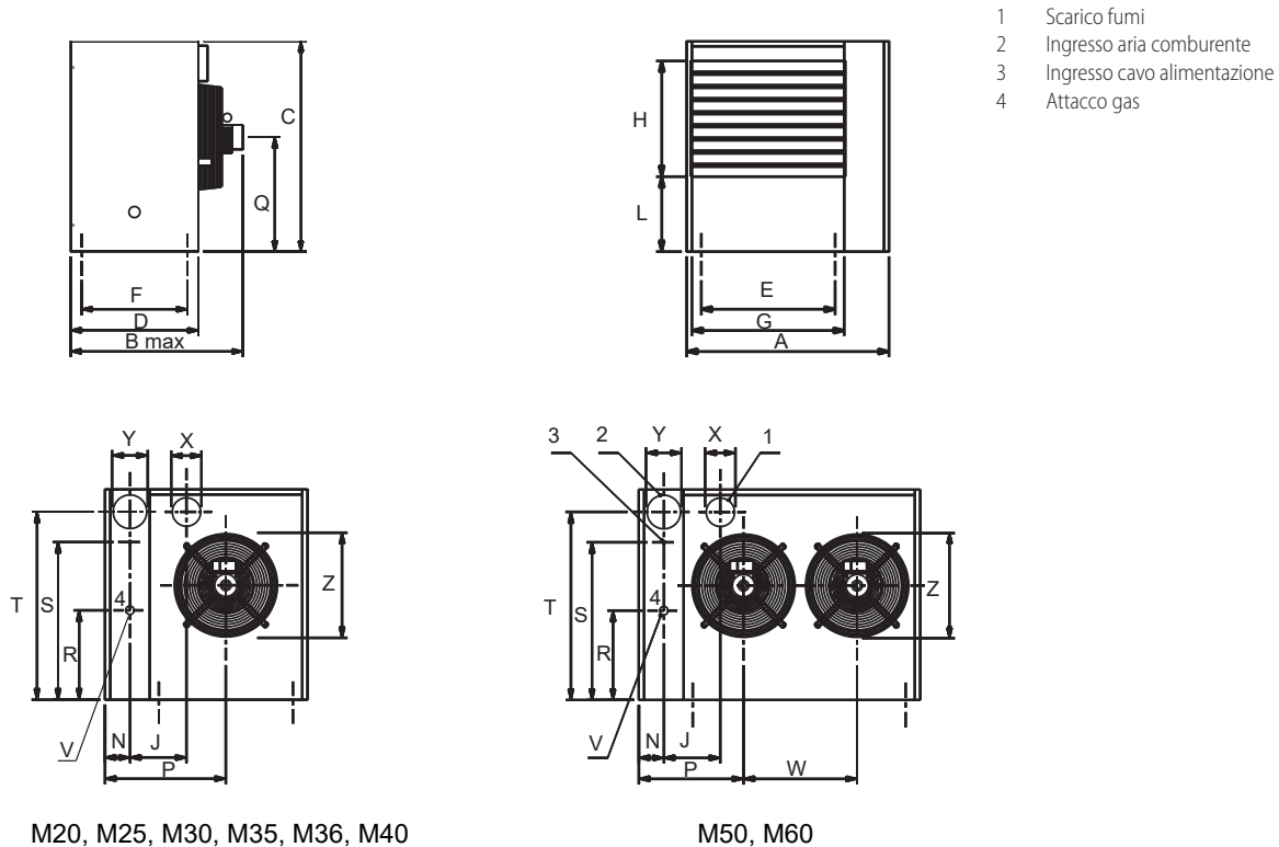
Figura 4.1 Dimensioni generatori serie M
